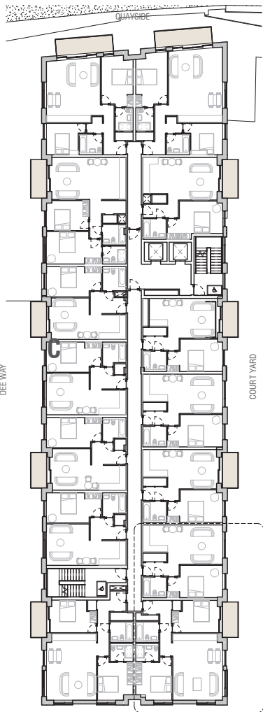
4 Block C - Level 05 1 : 200
